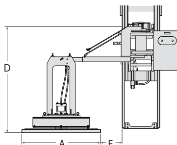
ステーションナリー サイドマウント (特殊マスト付)
