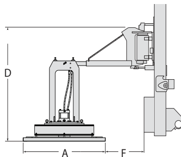
スイングモデル (特殊マスト付)
